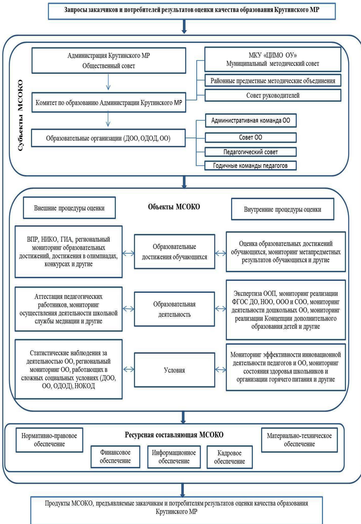
Рисунок 1. Модель МСОКО
